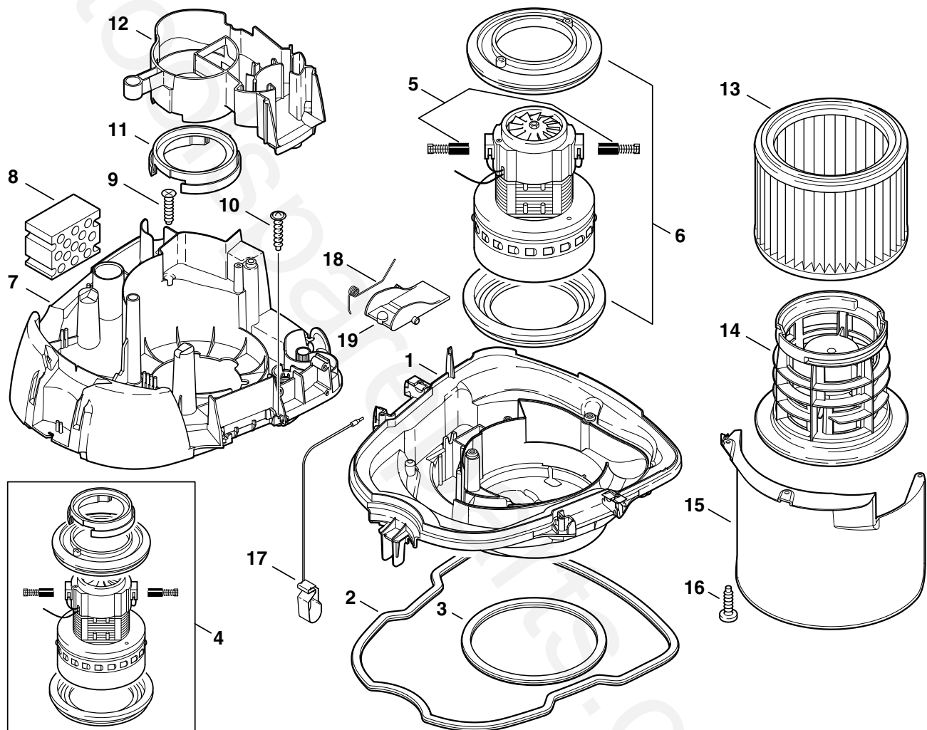
MAKITA 446L ( 3.12.2003)
